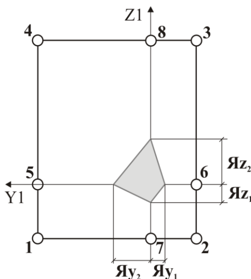
Рис. 6.2. Условное прямоугольное сечение
