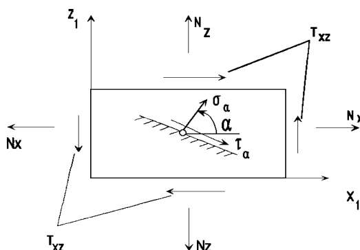
Рис. 6.3. Плоское напряженное состояние
